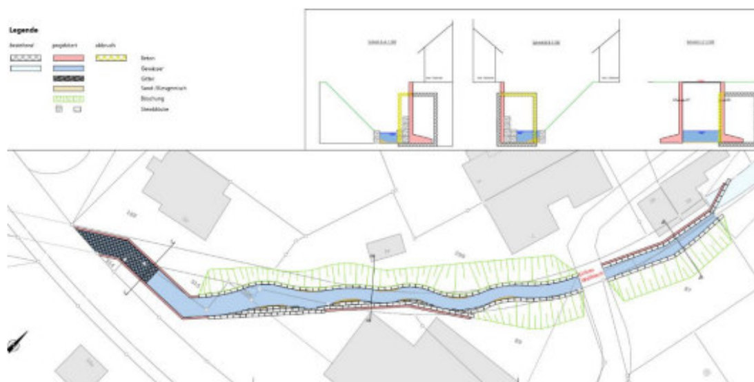
Abbildung 22: Ausschnitt aus dem Übersichtsplan Machbarkeitsstudie (Siehe Beilage).
